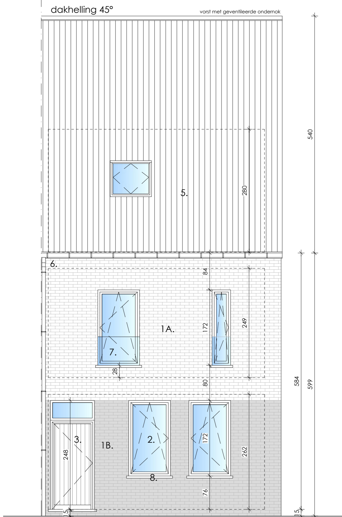
voorgevel woning C5
